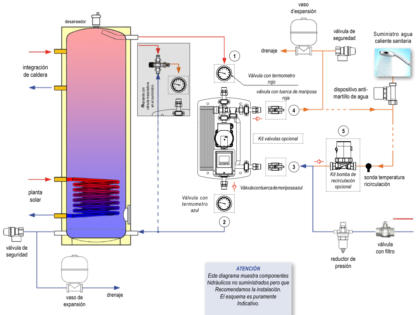
Figura 1: Esquema de una planta de ACS gestionada a través de ModvFresh 2
