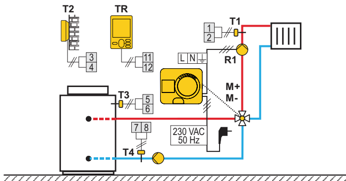
Diagrama 361 - Circuito de calefacción y regulación del retorno
